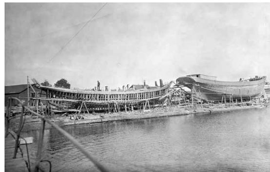
Kaksi kaljaasia rakenteilla Koivistolla vuonna 1914. Kuva: U. T. Sirelius, Museovirasto.
